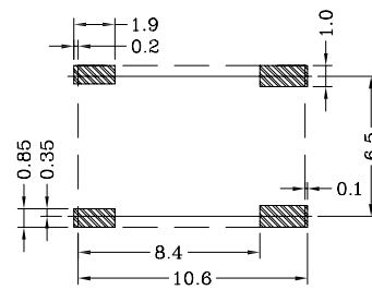
P.C.B. LAYOUT 线路板布局图
